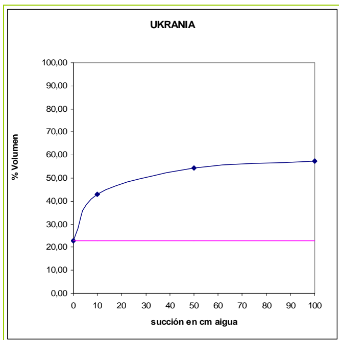
Curva de retención de agua. Elaboración propia.
